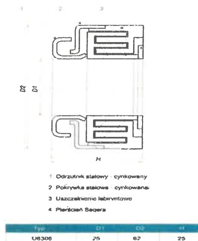
Uszczelnienie labiryntowe z odrzutnikiem
